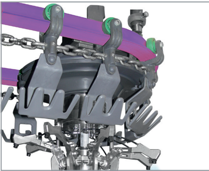
Kesimhane taşıma sistemleri için ray profilleri (mor renkli)
